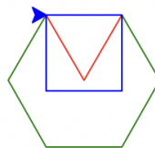
Programm 4.3: farb_vieleck.py
