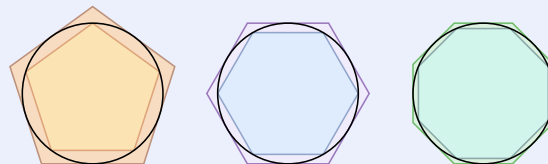
Abbildung 2.4: Schrittweise Annäherung an einen Kreis durch ein- beziehungsweise umschriebene regelmässige Polygone (links: 5-Ecke, Mitte: 6-Ecke, rechts: 8-Ecke).
