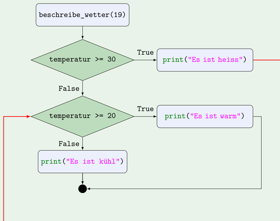
Abbildung 5.2: Flussdiagramm für den Code aus Aufgabe 5.6
